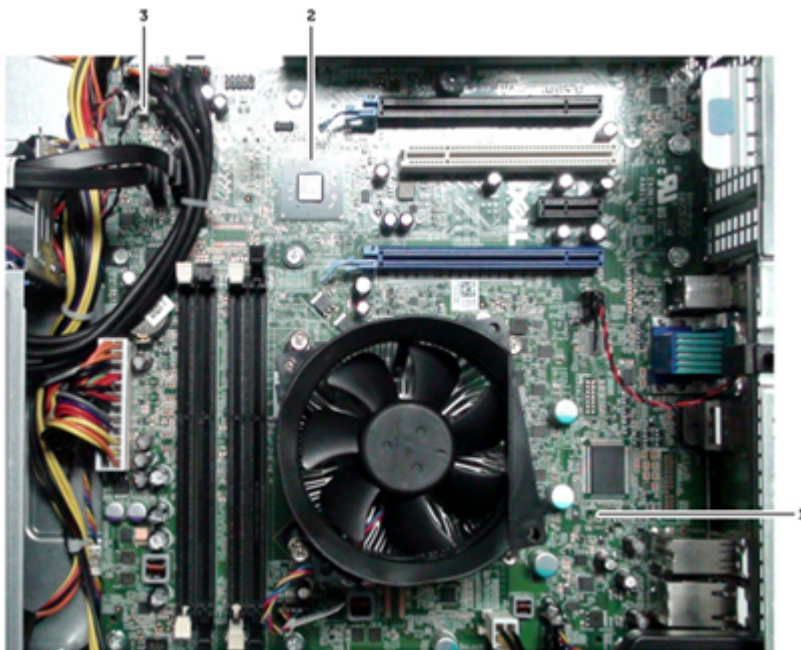
图 2: 拆下热传感器和散热器的系统板
